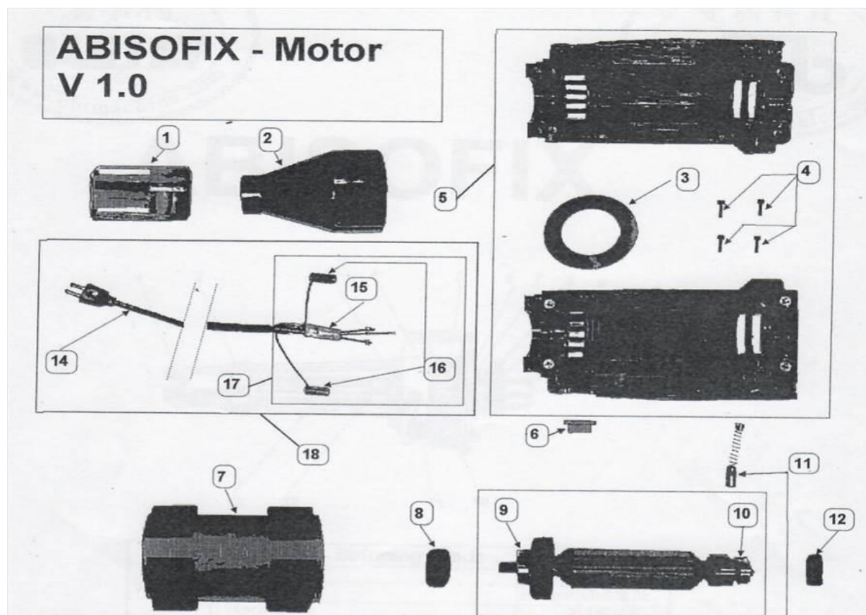
ABISOFIX - Motor Part List
